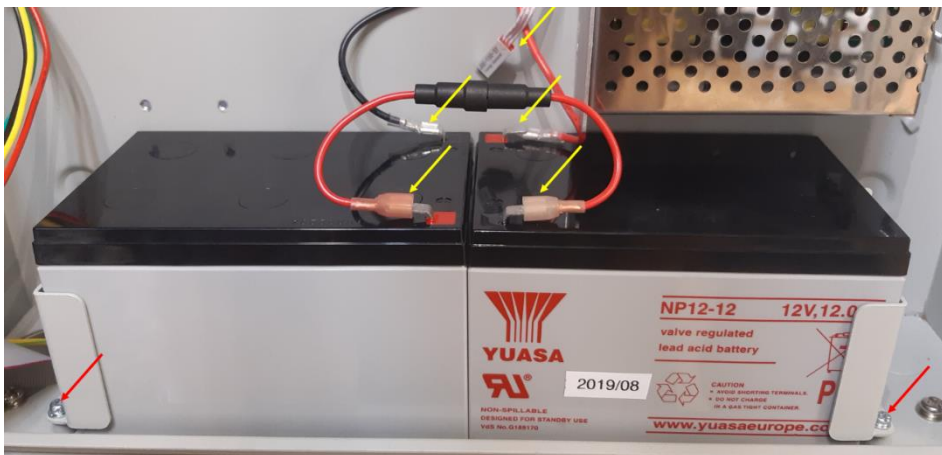
Figura 8: Ubicación de la conexión de la batería para 12 Ah
