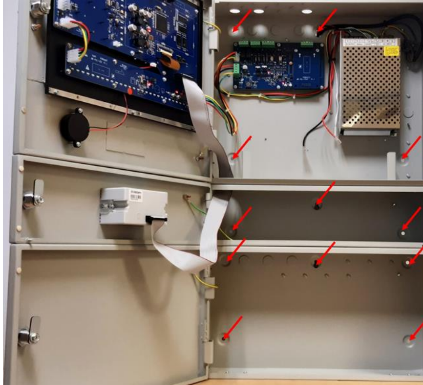
Figura 3: Ubicaciones de las perforaciones de montaje
